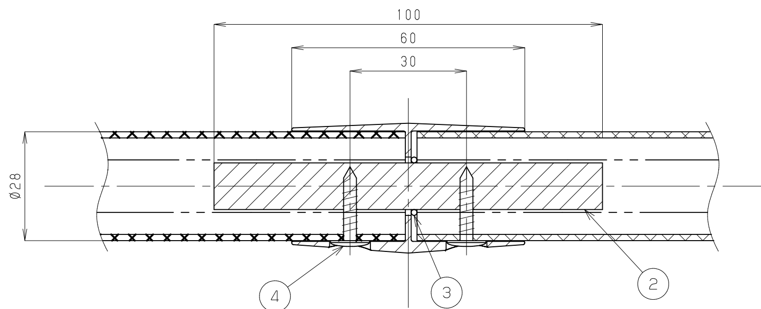
ビーム用ジョイント納まり図
